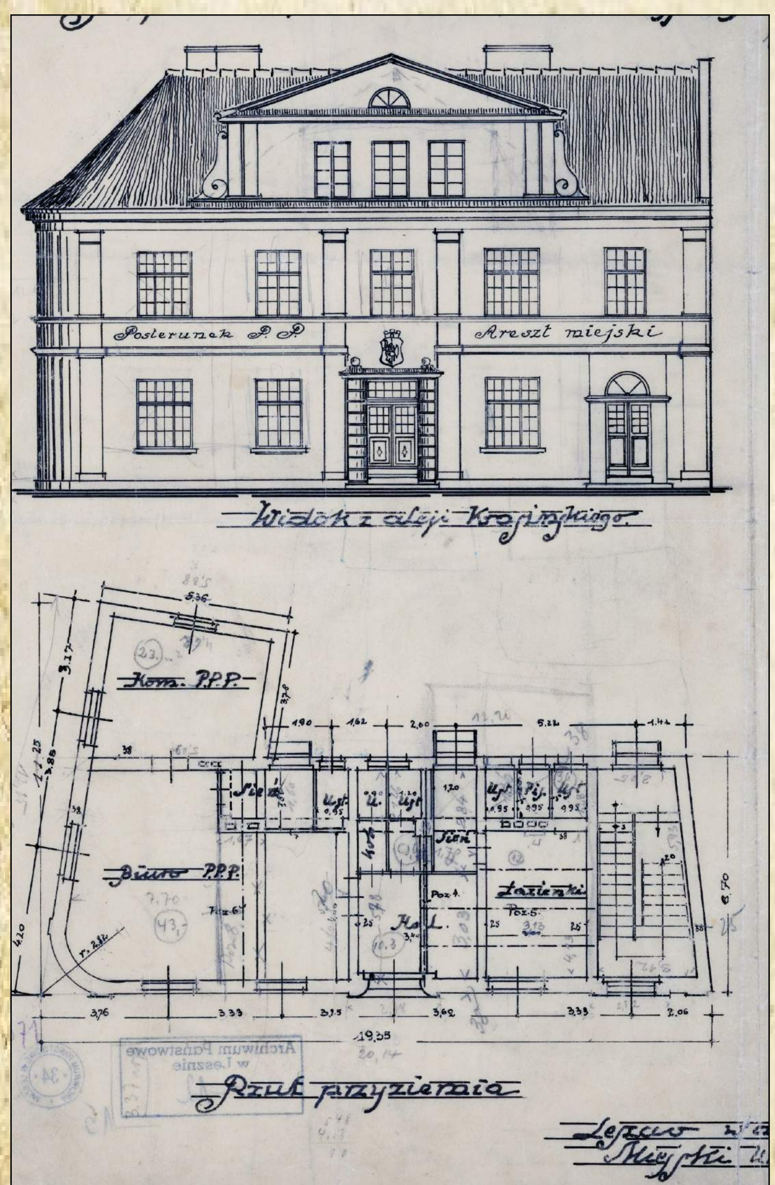
Projekt przebudowy więzienia miejskiego na areszt miejski i posterunek policji przy ul. Wałowej, czerwiec 1926 r.
